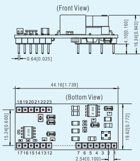
TLAxx-03K485 Series; LxWxH: 44.16x19.62x16.34(mm)
